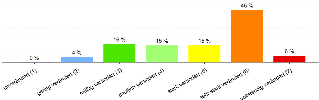
Abbildung 24: Anteil der Gewässerstrukturklassen im Wasserkörper DERW_DENW_3146_0_9: Beilbach
