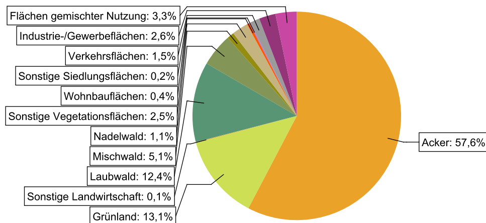
Abbildung 17: Landnutzung im Einzugsgebiet des Wasserkörpers DERW_DENW_31434_0_4: Klaverbach, basierend auf ATKIS-Daten 2024. Landnutzungstypen mit weniger als 0,1% Anteil sind nicht dargestellt.
