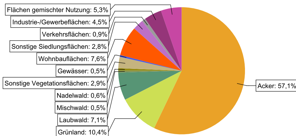
Abbildung 9: Landnutzung im Einzugsgebiet des Wasserkörpers DERW_DENW_314_26_34: Axtbach, basierend auf ATKIS-Daten 2024. Landnutzungstypen mit weniger als 0,1% Anteil sind nicht dargestellt.
