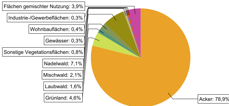
Abbildung 29: Landnutzung im Einzugsgebiet des Wasserkörpers DERW_DENW_31472_0_9: Flütbach, basierend auf ATKIS-Daten 2024. Landnutzungstypen mit weniger als 0,1% Anteil sind nicht dargestellt.
