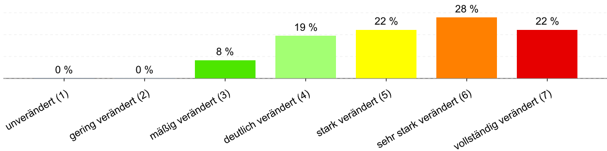
Abbildung 14: Anteil der Gewässerstrukturklassen im Wasserkörper DERW_DENW_3142_0_4: Bergeler Bach
