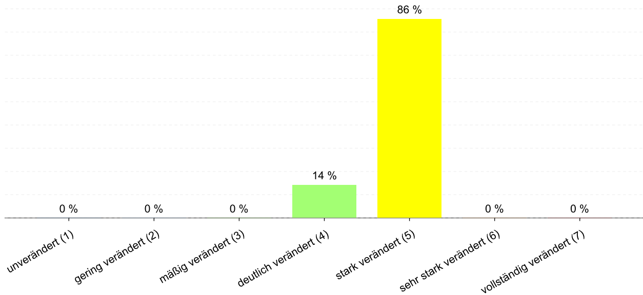
Abbildung 40: Anteil der Gewässerstrukturklassen im Wasserkörper DERW_DENW_3172_0_8: Mussenbach
