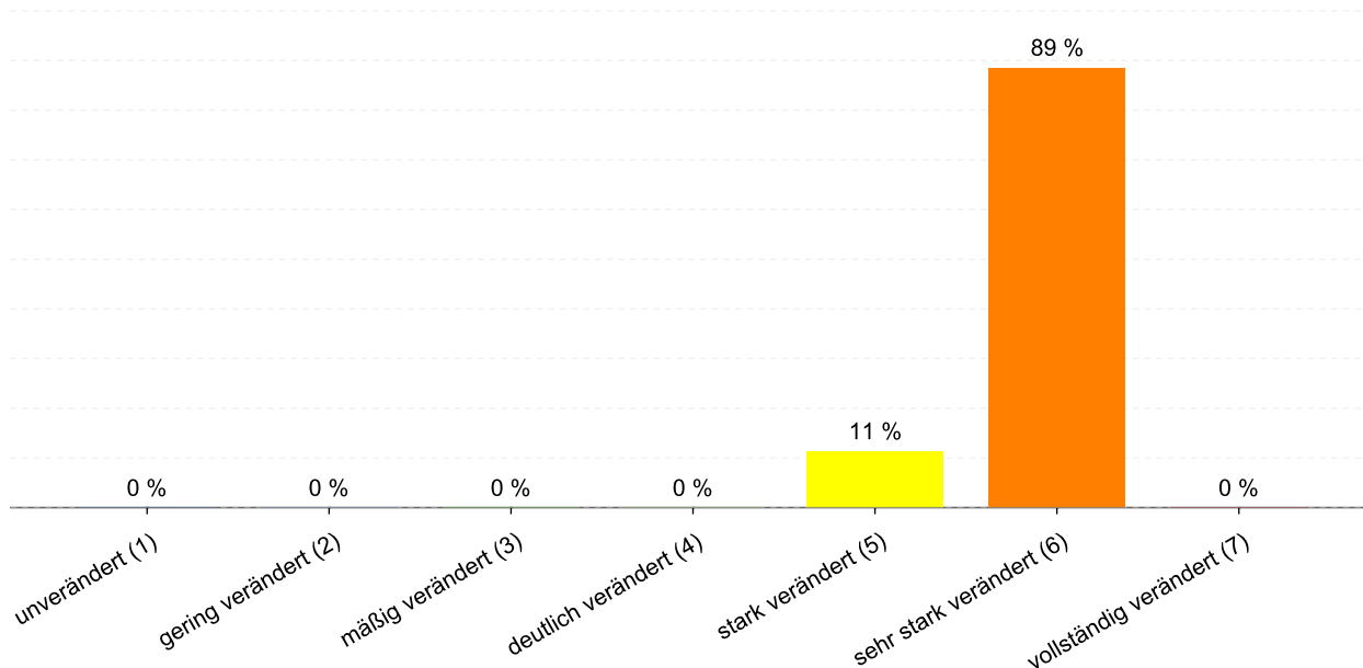
Abbildung 20: Anteil der Gewässerstrukturklassen im Wasserkörper DERW_DENW_3144_0_4: Maibach
