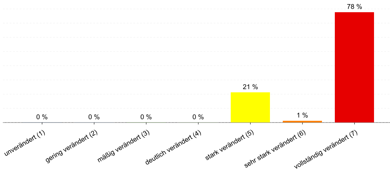
Abbildung 32: Anteil der Gewässerstrukturklassen im Wasserkörper DERW_DENW_3148_0_9: Baarbach
