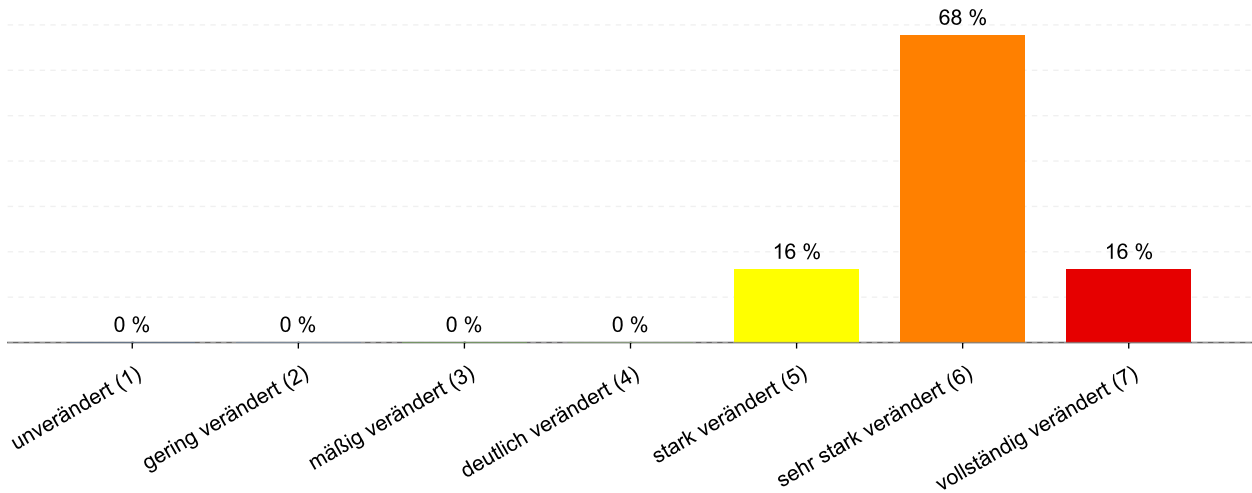
Abbildung 22: Anteil der Gewässerstrukturklassen im Wasserkörper DERW_DENW_3144_4_8: Maibach
