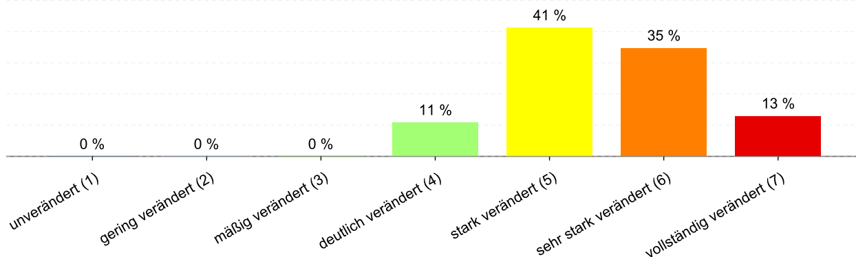
Abbildung 34: Anteil der Gewässerstrukturklassen im Wasserkörper DERW_DENW_3148_9_13: Mühlenbach
