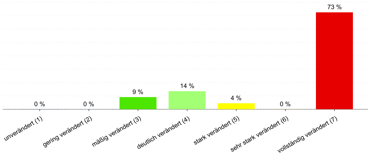
Abbildung 44: Anteil der Gewässerstrukturklassen im Wasserkörper DERW_DENW_31722_0_2: Brüggelbach
