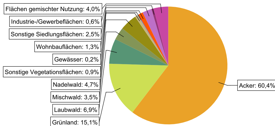
Abbildung 31: Landnutzung im Einzugsgebiet des Wasserkörpers DERW_DENW_3148_0_9: Baarbach, basierend auf ATKIS-Daten 2024. Landnutzungstypen mit weniger als 0,1% Anteil sind nicht dargestellt.
