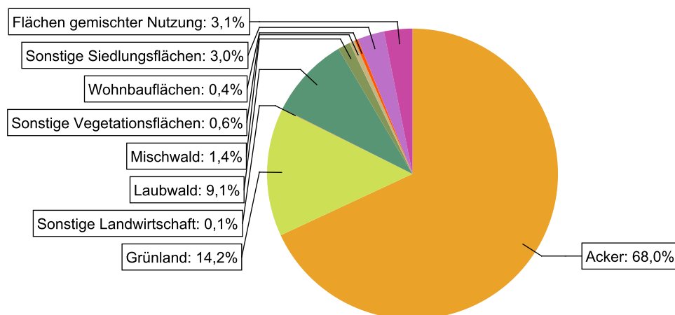
Abbildung 41: Landnutzung im Einzugsgebiet des Wasserkörpers DERW_DENW_3172_8_24: Mussenbach, basierend auf ATKIS-Daten 2024. Landnutzungstypen mit weniger als 0,1% Anteil sind nicht dargestellt.
