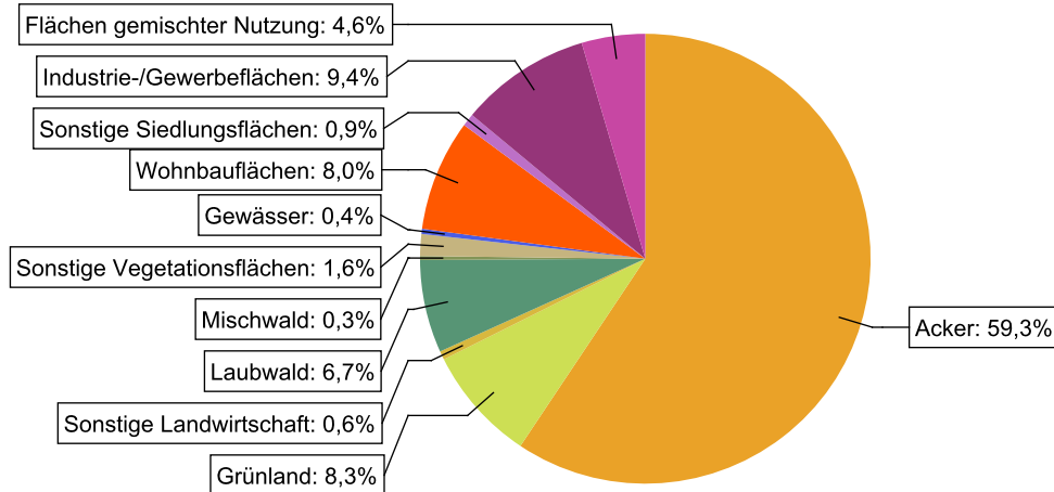
Abbildung 33: Landnutzung im Einzugsgebiet des Wasserkörpers DERW_DENW_3148_9_13: Mühlenbach, basierend auf ATKIS-Daten 2024. Landnutzungstypen mit weniger als 0,1% Anteil sind nicht dargestellt.
