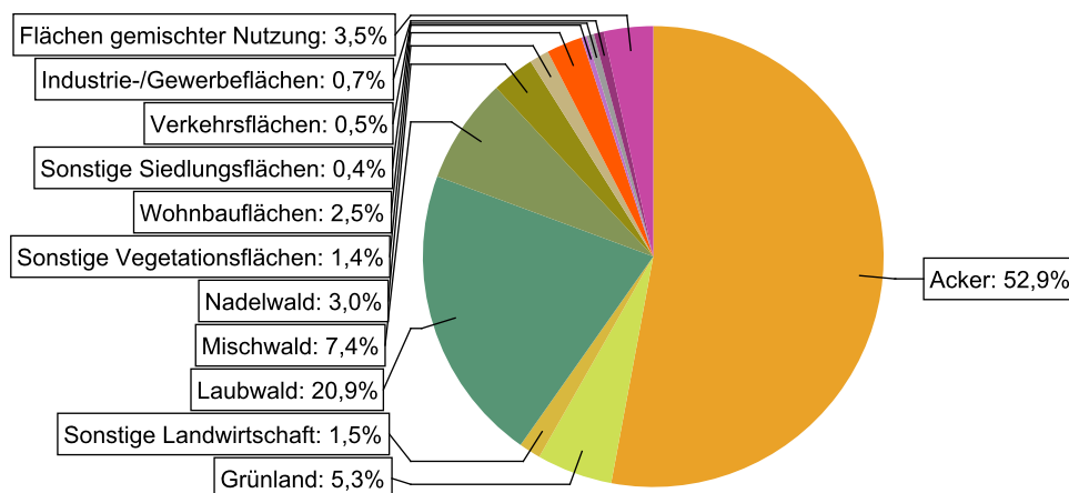
Abbildung 15: Landnutzung im Einzugsgebiet des Wasserkörpers DERW_DENW_3142_4_8: Bergeler Bach, basierend auf ATKIS-Daten 2024. Landnutzungstypen mit weniger als 0,1% Anteil sind nicht dargestellt.
