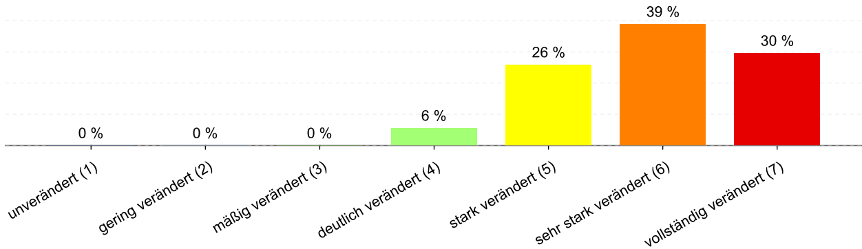
Abbildung 8: Anteil der Gewässerstrukturklassen im Wasserkörper DERW_DENW_314_21_26: Axtbach
