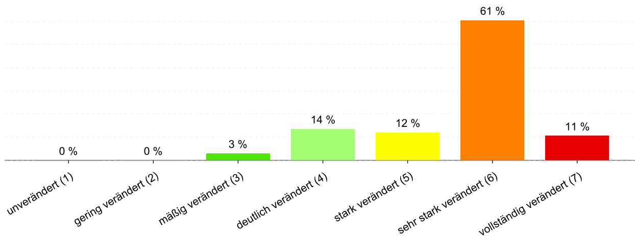
Abbildung 12: Anteil der Gewässerstrukturklassen im Wasserkörper DERW_DENW_31414_0_6: Stichelbach
