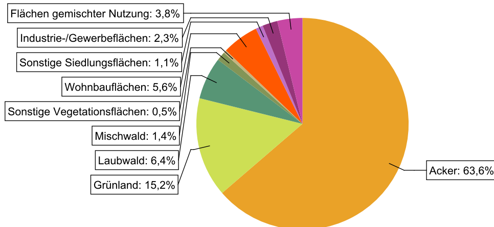
Abbildung 45: Landnutzung im Einzugsgebiet des Wasserkörpers DERW_DENW_31722_2_12: Brüggenbach, basierend auf ATKIS-Daten 2024. Landnutzungstypen mit weniger als 0,1% Anteil sind nicht dargestellt.
