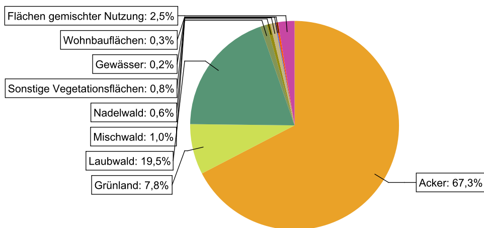
Abbildung 25: Landnutzung im Einzugsgebiet des Wasserkörpers DERW_DENW_3146_9_15: Beilbach, basierend auf ATKIS-Daten 2024. Landnutzungstypen mit weniger als 0,1% Anteil sind nicht dargestellt.
