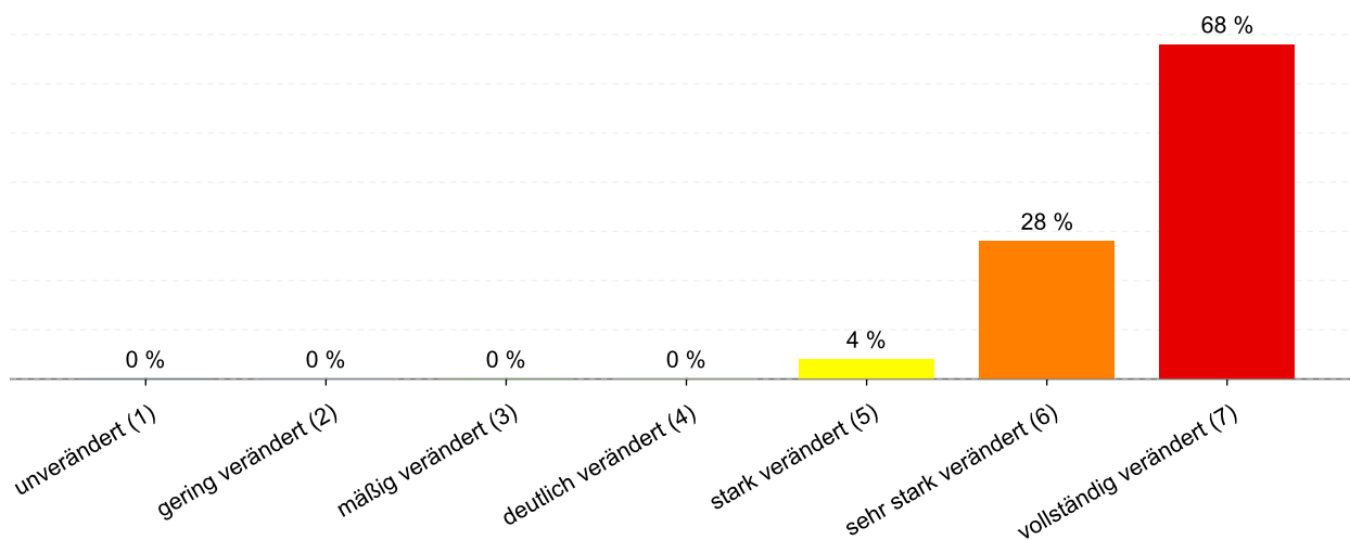
Abbildung 38: Anteil der Gewässerstrukturklassen im Wasserkörper DERW_DENW_3154_9_11: Holzbach
