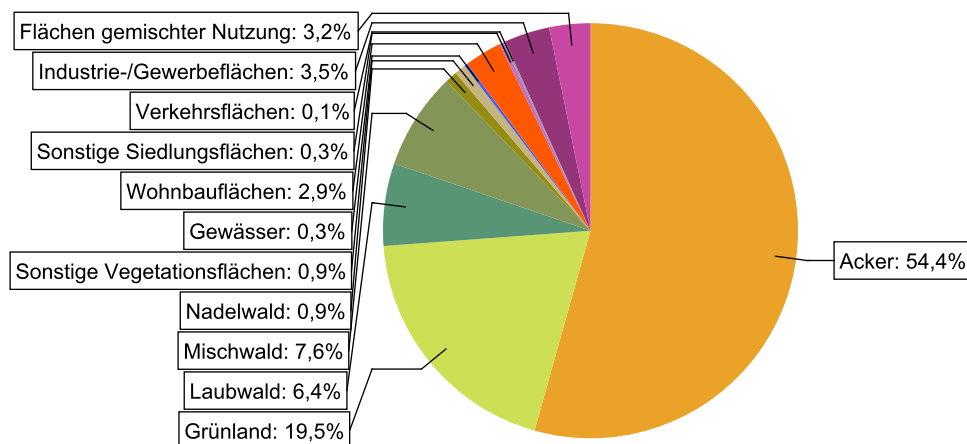
Abbildung 35: Landnutzung im Einzugsgebiet des Wasserkörpers DERW_DENW_3154_0_9: Holzbach, basierend auf ATKIS-Daten 2024. Landnutzungstypen mit weniger als 0,1% Anteil sind nicht dargestellt.
