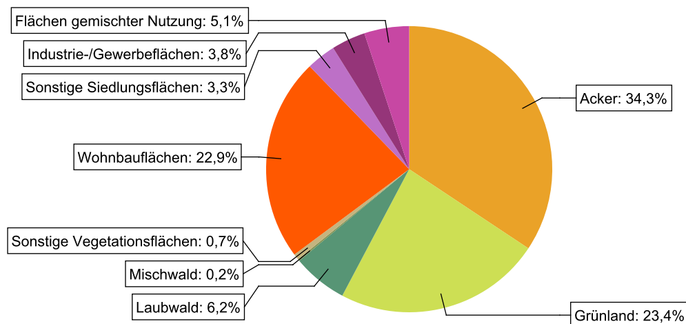
Abbildung 37: Landnutzung im Einzugsgebiet des Wasserkörpers DERW_DENW_3154_9_11: Holzbach, basierend auf ATKIS-Daten 2024. Landnutzungstypen mit weniger als 0,1% Anteil sind nicht dargestellt.
