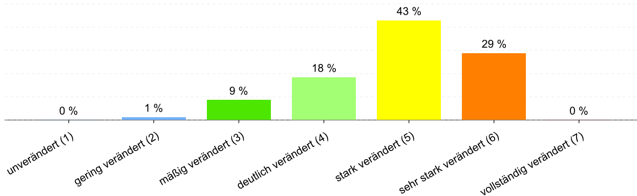
Abbildung 42: Anteil der Gewässerstrukturklassen im Wasserkörper DERW_DENW_3172_8_24: Mussenbach
