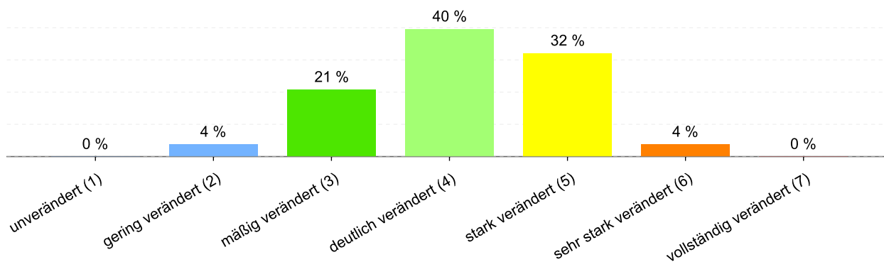
Abbildung 26: Anteil der Gewässerstrukturklassen im Wasserkörper DERW_DENW_3146_9_15: Beilbach
