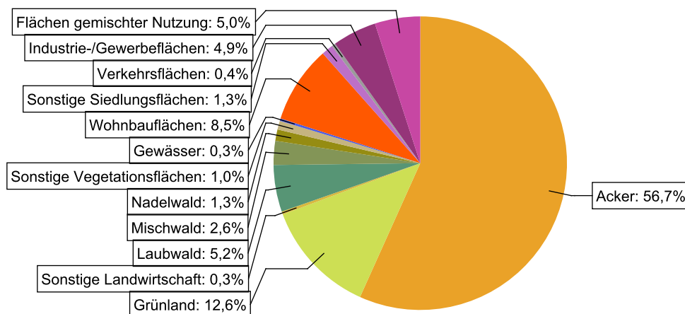
Abbildung 5: Landnutzung im Einzugsgebiet des Wasserkörpers DERW_DENW_314_7_21: Axtbach, basierend auf ATKIS-Daten 2024. Landnutzungstypen mit weniger als 0,1% Anteil sind nicht dargestellt.
