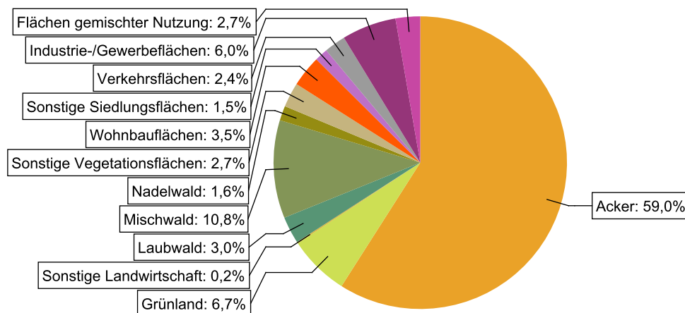
Abbildung 13: Landnutzung im Einzugsgebiet des Wasserkörpers DERW_DENW_3142_0_4: Bergeler Bach, basierend auf ATKIS-Daten 2024. Landnutzungstypen mit weniger als 0,1% Anteil sind nicht dargestellt.
