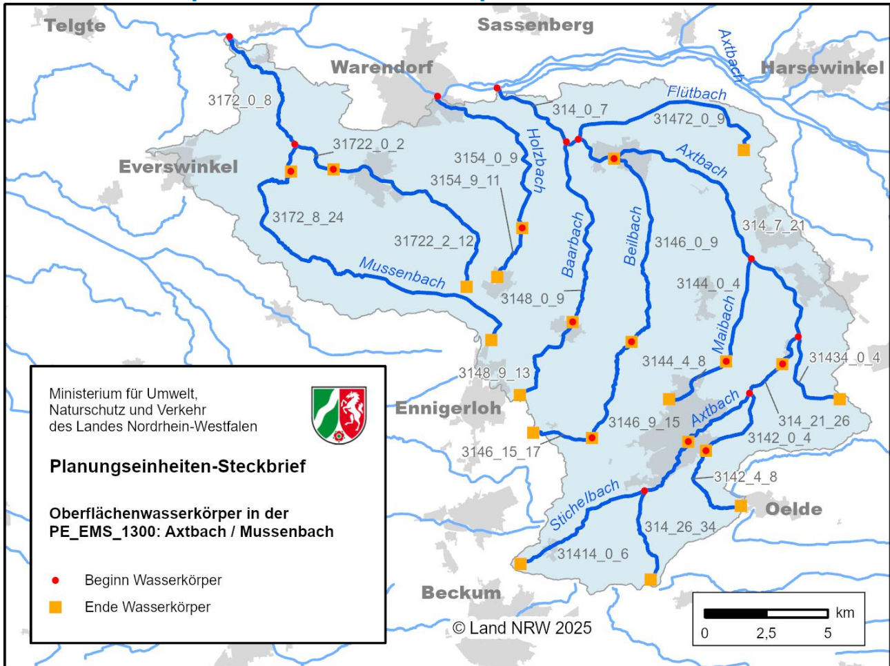
Abbildung 2: Oberflächenwasserkörper in der Planungseinheit PE_EMS_1300: Axtbach / Mussenbach
