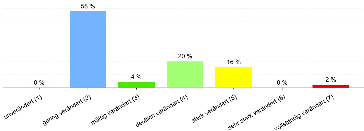
Abbildung 16: Anteil der Gewässerstrukturklassen im Wasserkörper DERW_DENW_3142_4_8: Bergeler Bach
