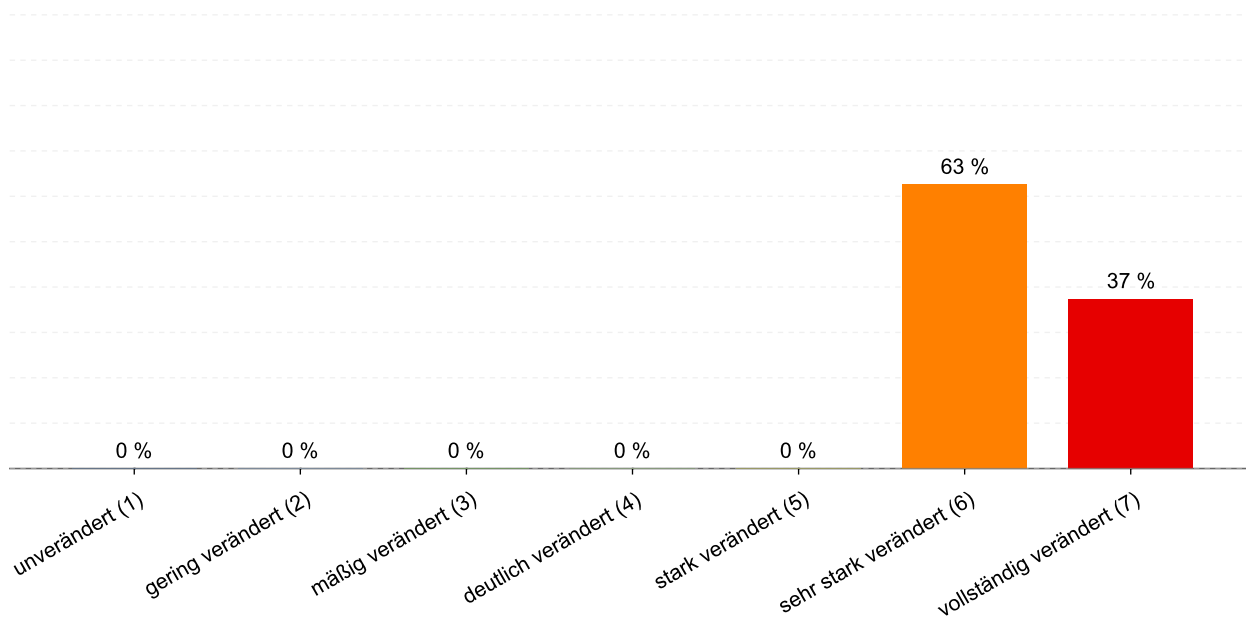
Abbildung 30: Anteil der Gewässerstrukturklassen im Wasserkörper DERW_DENW_31472_0_9: Flütbach
