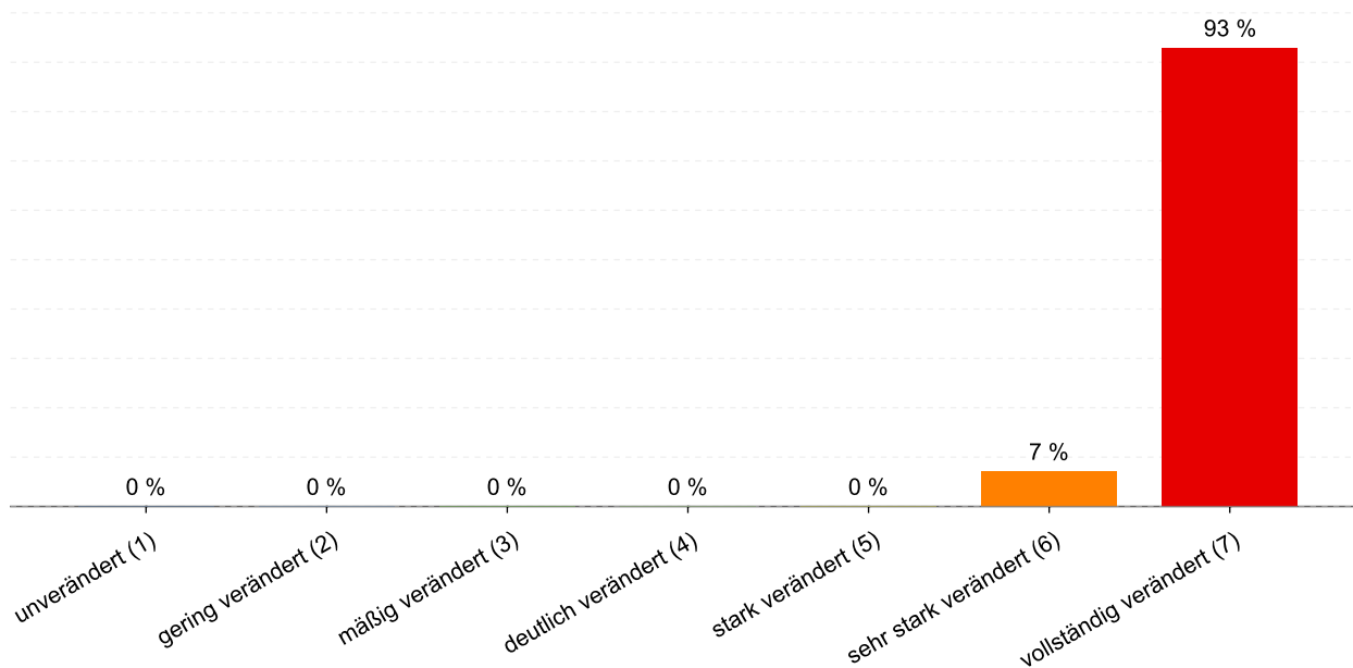
Abbildung 18: Anteil der Gewässerstrukturklassen im Wasserkörper DERW_DENW_31434_0_4: Klaverbach
