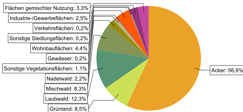
Abbildung 39: Landnutzung im Einzugsgebiet des Wasserkörpers DERW_DENW_3172_0_8: Mussenbach, basierend auf ATKIS-Daten 2024. Landnutzungstypen mit weniger als 0,1% Anteil sind nicht dargestellt.
