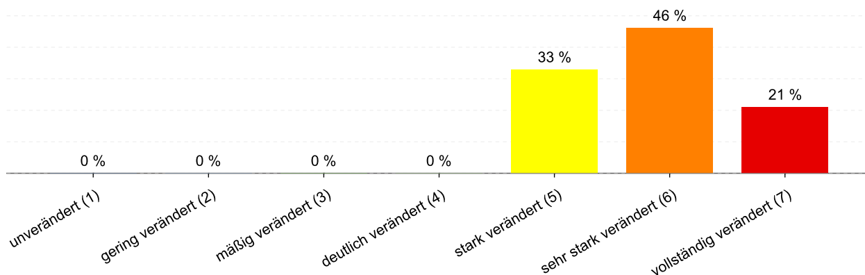
Abbildung 6: Anteil der Gewässerstrukturklassen im Wasserkörper DERW_DENW_314_7_21: Axtbach
