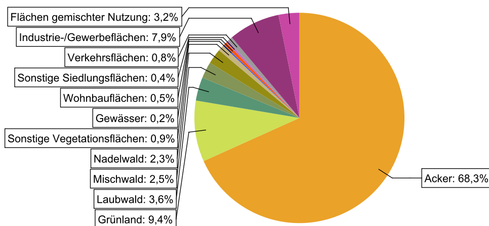
Abbildung 3: Landnutzung im Einzugsgebiet des Wasserkörpers DERW_DENW_314_0_7: Axtbach, basierend auf ATKIS-Daten 2024. Landnutzungstypen mit weniger als 0,1% Anteil sind nicht dargestellt.
