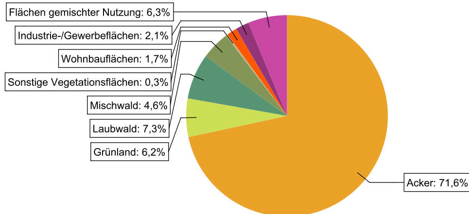
Abbildung 19: Landnutzung im Einzugsgebiet des Wasserkörpers DERW_DENW_3144_0_4: Maibach, basierend auf ATKIS-Daten 2024. Landnutzungstypen mit weniger als 0,1% Anteil sind nicht dargestellt.
