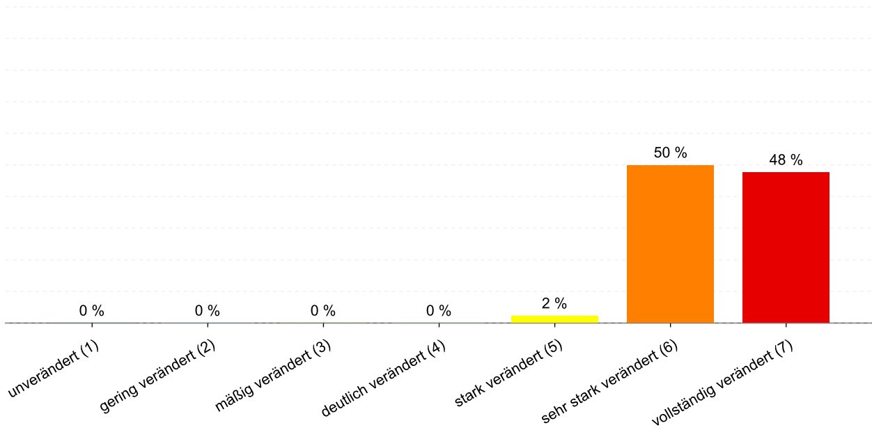
Abbildung 36: Anteil der Gewässerstrukturklassen im Wasserkörper DERW_DENW_3154_0_9: Holzbach
