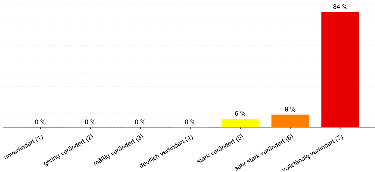
Abbildung 46: Anteil der Gewässerstrukturklassen im Wasserkörper DERW_DENW_31722_2_12: Brüggelbach
