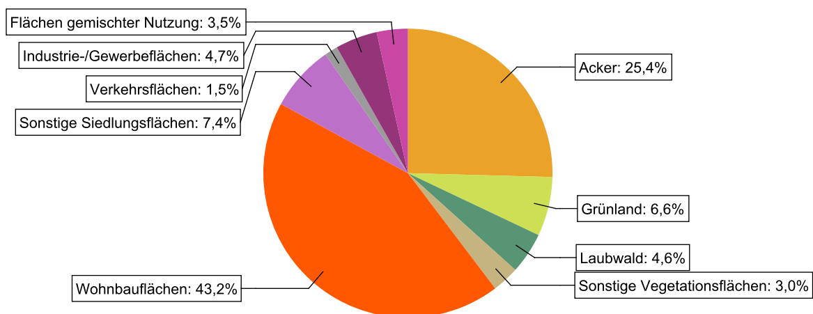
Abbildung 7: Landnutzung im Einzugsgebiet des Wasserkörpers DERW_DENW_314_21_26: Axtbach, basierend auf ATKIS-Daten 2024. Landnutzungstypen mit weniger als 0,1% Anteil sind nicht dargestellt.
