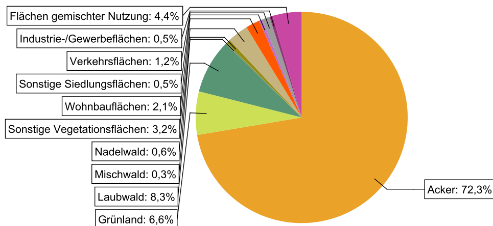
Abbildung 11: Landnutzung im Einzugsgebiet des Wasserkörpers DERW_DENW_31414_0_6: Stichelbach, basierend auf ATKIS-Daten 2024. Landnutzungstypen mit weniger als 0,1% Anteil sind nicht dargestellt.
