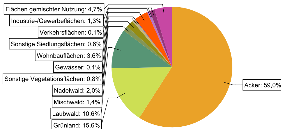
Abbildung 23: Landnutzung im Einzugsgebiet des Wasserkörpers DERW_DENW_3146_0_9: Beilbach, basierend auf ATKIS-Daten 2024. Landnutzungstypen mit weniger als 0,1% Anteil sind nicht dargestellt.
