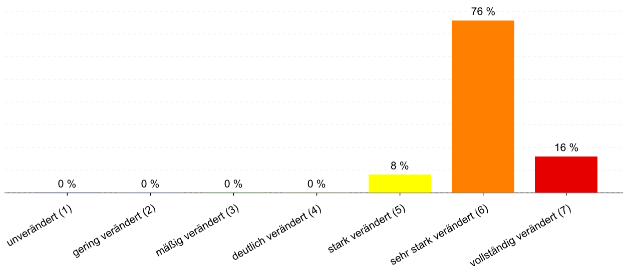
Abbildung 28: Anteil der Gewässerstrukturklassen im Wasserkörper DERW_DENW_3146_15_17: Merscbach
