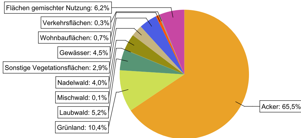
Abbildung 27: Landnutzung im Einzugsgebiet des Wasserkörpers DERW_DENW_3146_15_17: Merschbach, basierend auf ATKIS-Daten 2024. Landnutzungstypen mit weniger als 0,1% Anteil sind nicht dargestellt.
