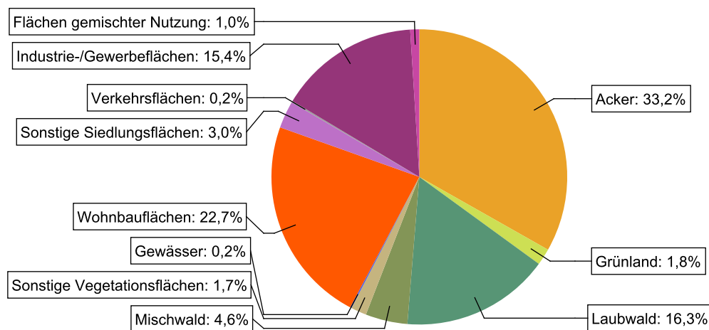
Abbildung 21: Landnutzung im Einzugsgebiet des Wasserkörpers DERW_DENW_3144_4_8: Maibach, basierend auf ATKIS-Daten 2024. Landnutzungstypen mit weniger als 0,1% Anteil sind nicht dargestellt.
