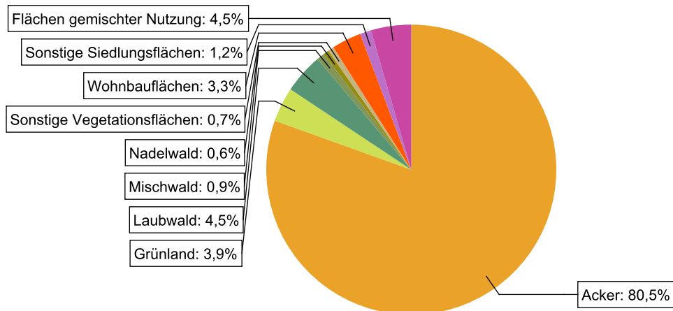
Abbildung 43: Landnutzung im Einzugsgebiet des Wasserkörpers DERW_DENW_31722_0_2: Brüggenbach, basierend auf ATKIS-Daten 2024. Landnutzungstypen mit weniger als 0,1% Anteil sind nicht dargestellt.
