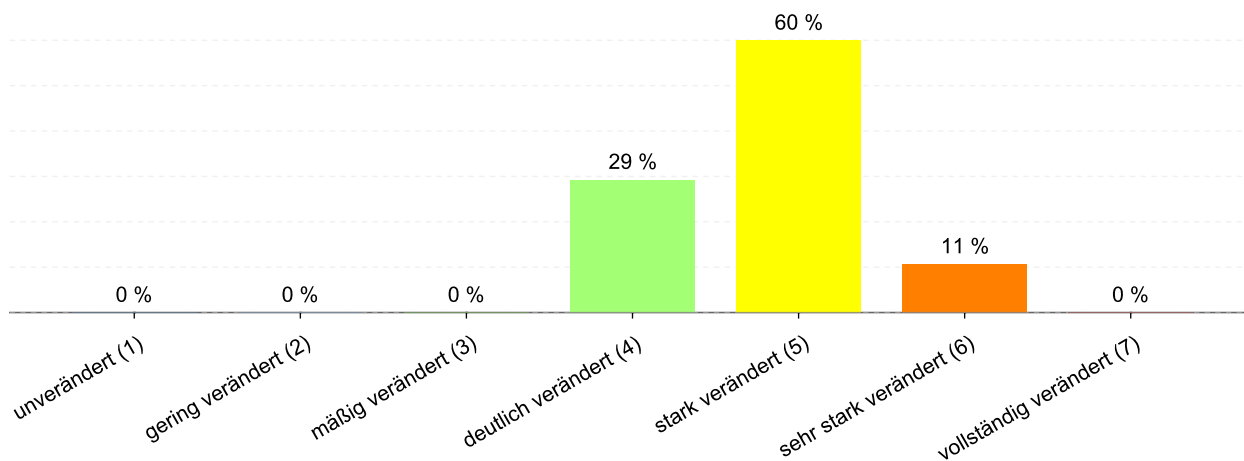
Abbildung 10: Anteil der Gewässerstrukturklassen im Wasserkörper DERW_DENW_314_26_34: Axtbach
