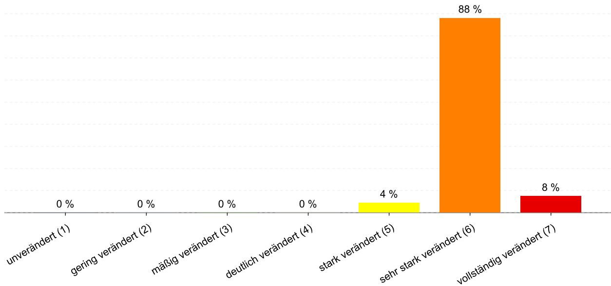
Abbildung 4: Anteil der Gewässerstrukturklassen im Wasserkörper DERW_DENW_314_0_7: Axtbach
