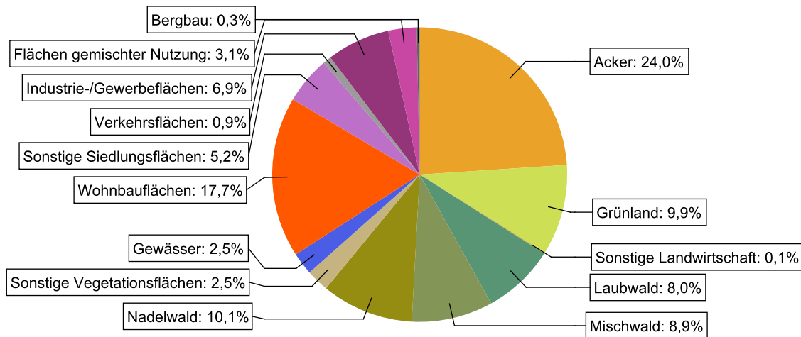
Abbildung 3: Landnutzung im Einzugsgebiet des Wasserkörpers DERW_DENW_27888_0_9: Halterner Mühlenbach, basierend auf ATKIS-Daten 2024. Landnutzungstypen mit weniger als 0,1% Anteil sind nicht dargestellt.
