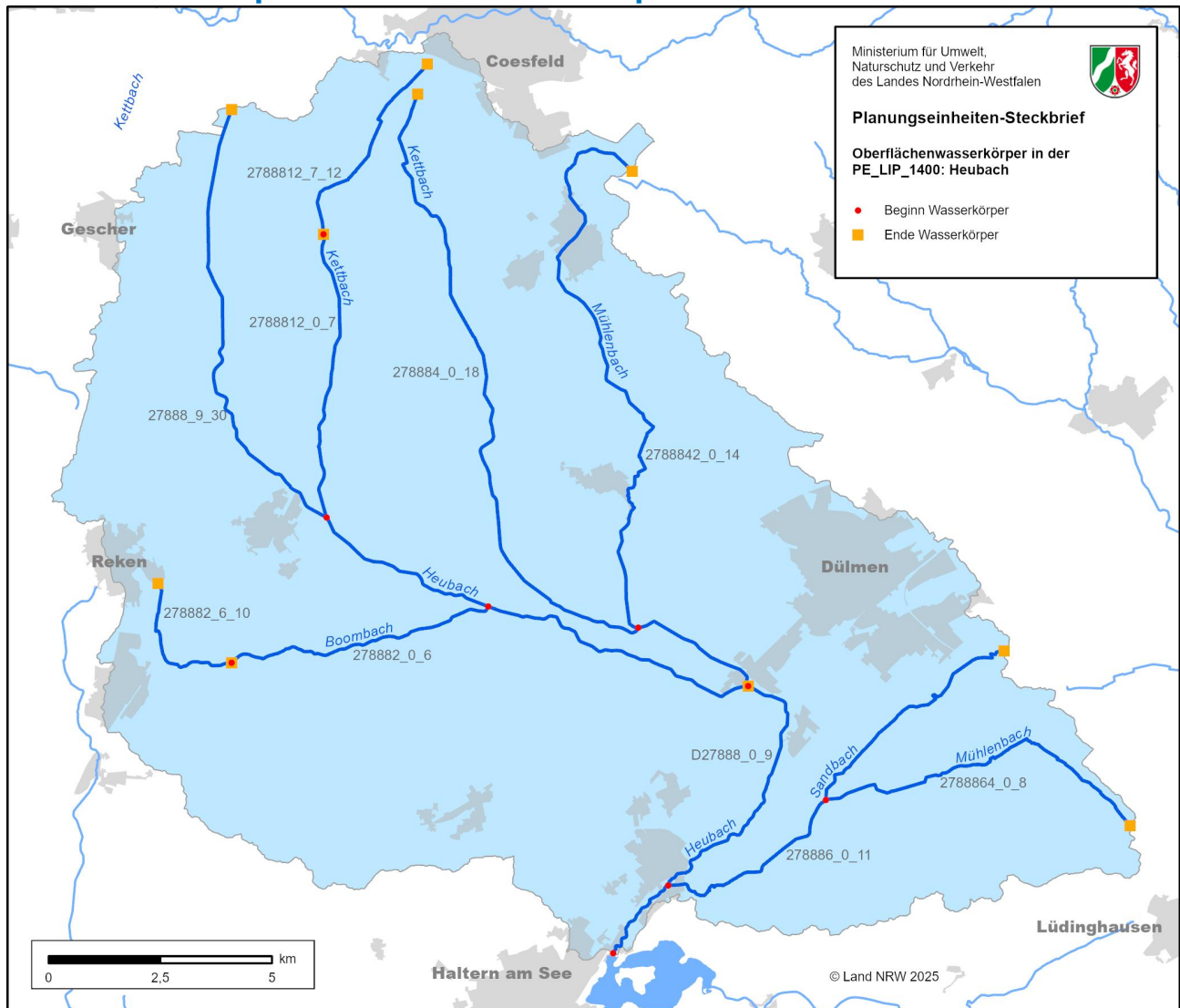
Abbildung 2: Oberflächenwasserkörper in der Planungseinheit PE_LIP_1400: Heubach
