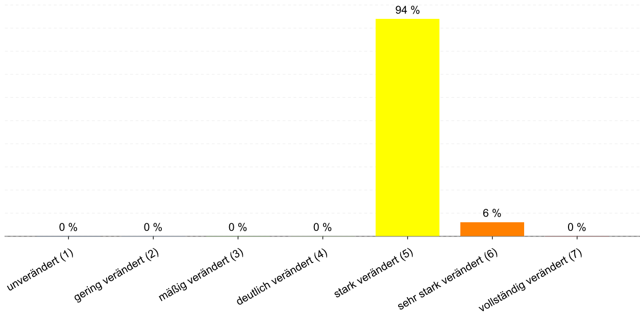
Abbildung 6: Anteil der Gewässerstrukturklassen im Wasserkörper DERW_DENW_27888_9_30: Heubach
