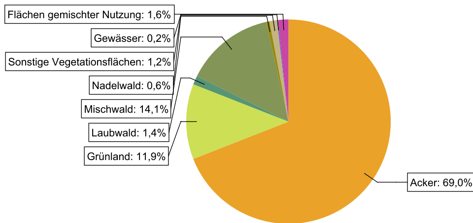
Abbildung 7: Landnutzung im Einzugsgebiet des Wasserkörpers DERW_DENW_2788812_0_7: Kettbach, basierend auf ATKIS-Daten 2024. Landnutzungstypen mit weniger als 0,1% Anteil sind nicht dargestellt.
