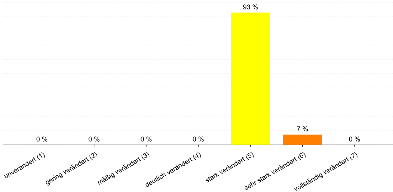
Abbildung 16: Anteil der Gewässerstrukturklassen im Wasserkörper DERW_DENW_278884_0_18: Kannebrocksbach
