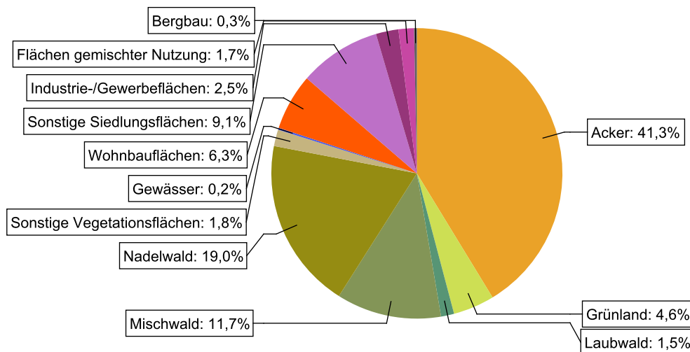
Abbildung 9: Landnutzung im Einzugsgebiet des Wasserkörpers DERW_DENW_2788812_7_12: Wienhörsterbach, basierend auf ATKIS-Daten 2024. Landnutzungstypen mit weniger als 0,1% Anteil sind nicht dargestellt.
