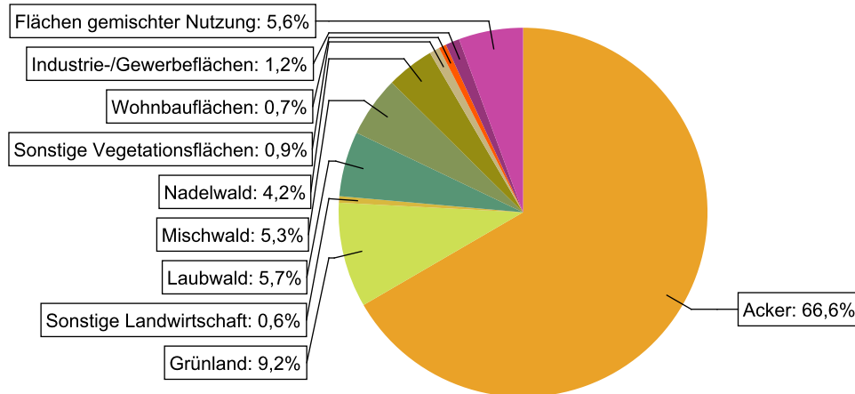
Abbildung 21: Landnutzung im Einzugsgebiet des Wasserkörpers DERW_DENW_2788864_0_8: Mühlenbach, basierend auf ATKIS-Daten 2024. Landnutzungstypen mit weniger als 0,1% Anteil sind nicht dargestellt.
