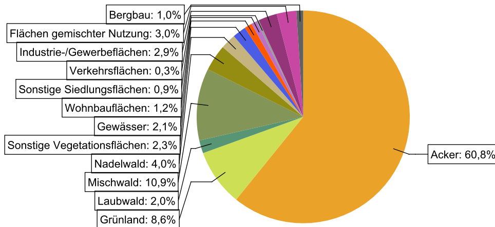
Abbildung 15: Landnutzung im Einzugsgebiet des Wasserkörpers DERW_DENW_278884_0_18: Kannebrocksbach, basierend auf ATKIS-Daten 2024. Landnutzungstypen mit weniger als 0,1% Anteil sind nicht dargestellt.
