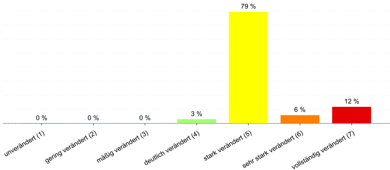
Abbildung 14: Anteil der Gewässerstrukturklassen im Wasserkörper DERW_DENW_278882_6_10: Boombach
