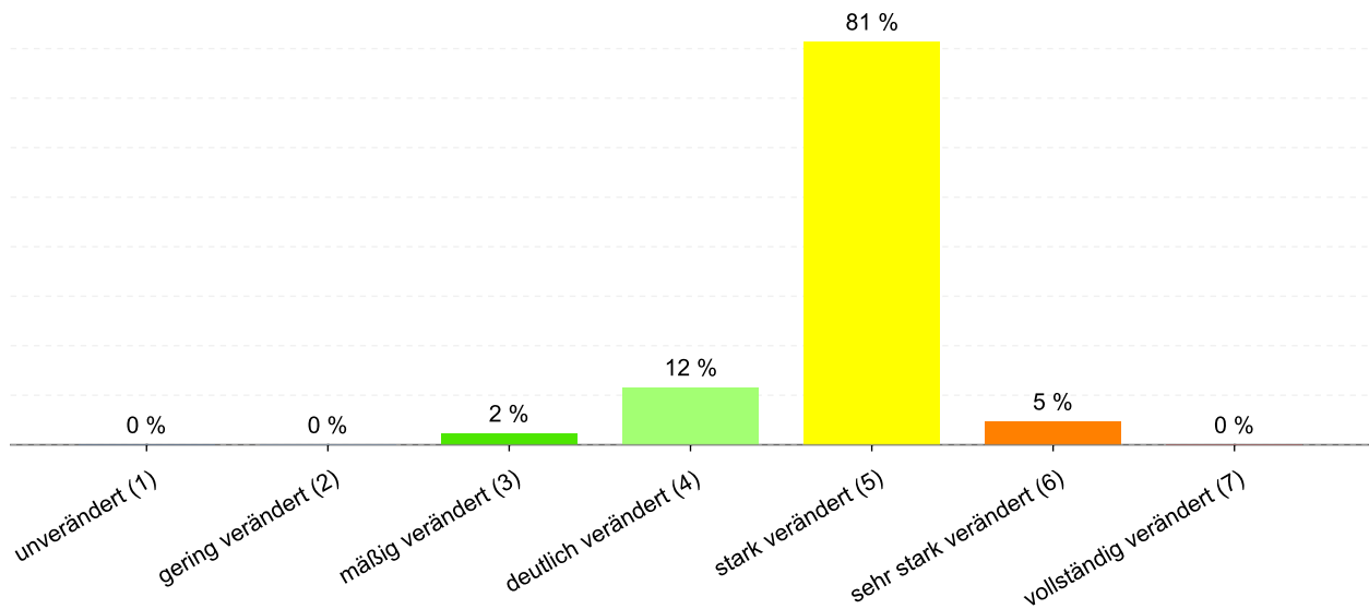
Abbildung 4: Anteil der Gewässerstrukturklassen im Wasserkörper DERW_DENW_27888_0_9: Halterner Mühlenbach
