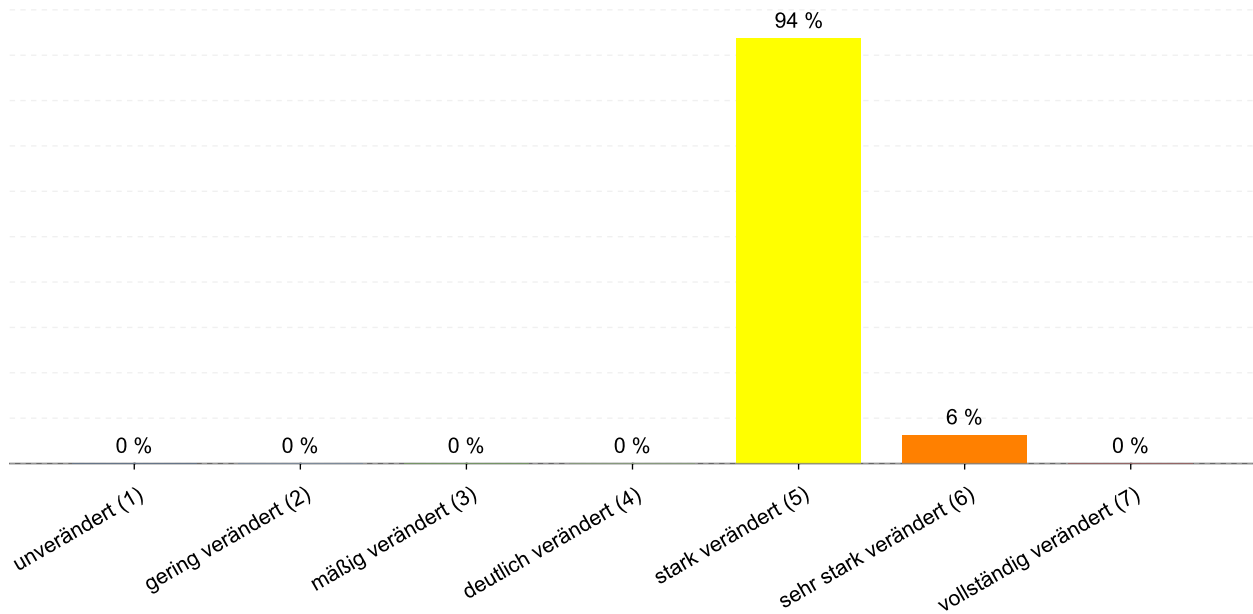
Abbildung 12: Anteil der Gewässerstrukturklassen im Wasserkörper DERW_DENW_278882_0_6: Boombach
