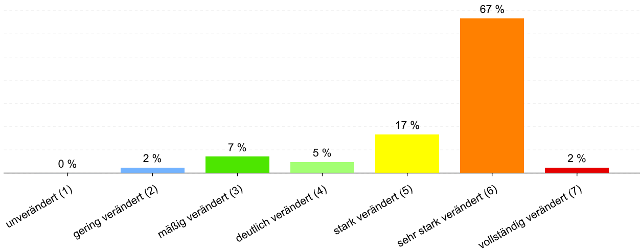
Abbildung 22: Anteil der Gewässerstrukturklassen im Wasserkörper DERW_DENW_2788864_0_8: Mühlenbach
