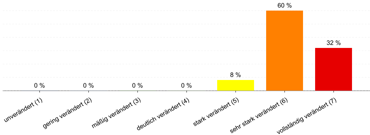
Abbildung 10: Anteil der Gewässerstrukturklassen im Wasserkörper DERW_DENW_2788812_7_12: Wienhörsterbach
