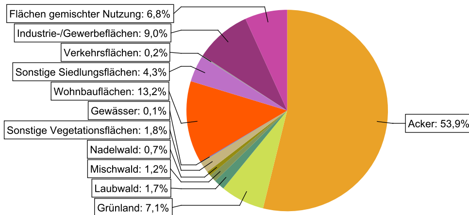
Abbildung 13: Landnutzung im Einzugsgebiet des Wasserkörpers DERW_DENW_278882_6_10: Boombach, basierend auf ATKIS-Daten 2024. Landnutzungstypen mit weniger als 0,1% Anteil sind nicht dargestellt.
