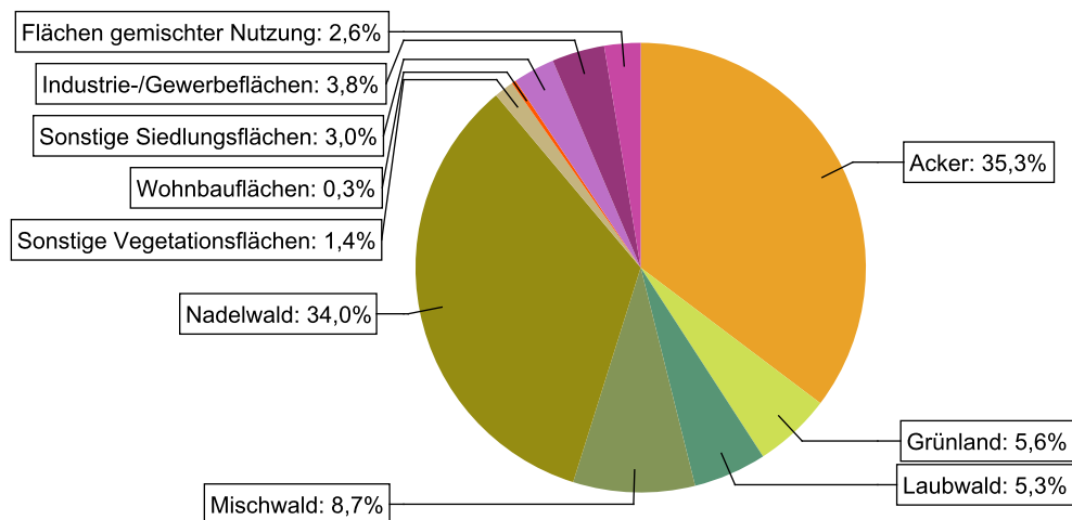
Abbildung 11: Landnutzung im Einzugsgebiet des Wasserkörpers DERW_DENW_278882_0_6: Boombach, basierend auf ATKIS-Daten 2024. Landnutzungstypen mit weniger als 0,1% Anteil sind nicht dargestellt.
