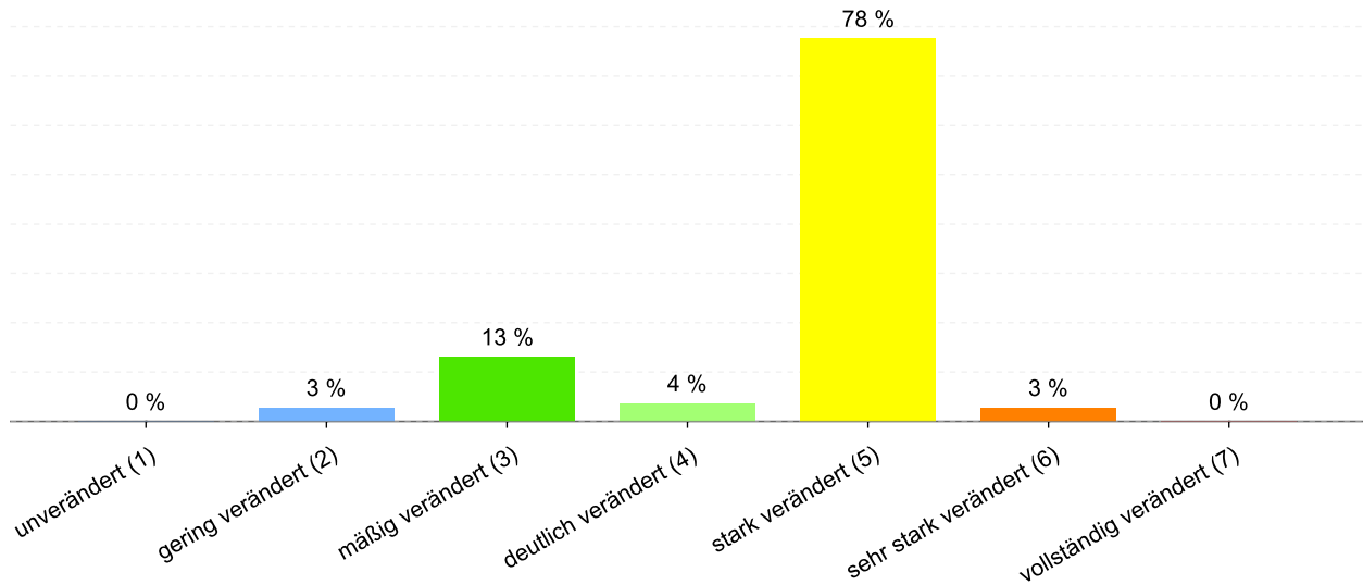
Abbildung 20: Anteil der Gewässerstrukturklassen im Wasserkörper DERW_DENW_278886_0_11: Kiffertbach
