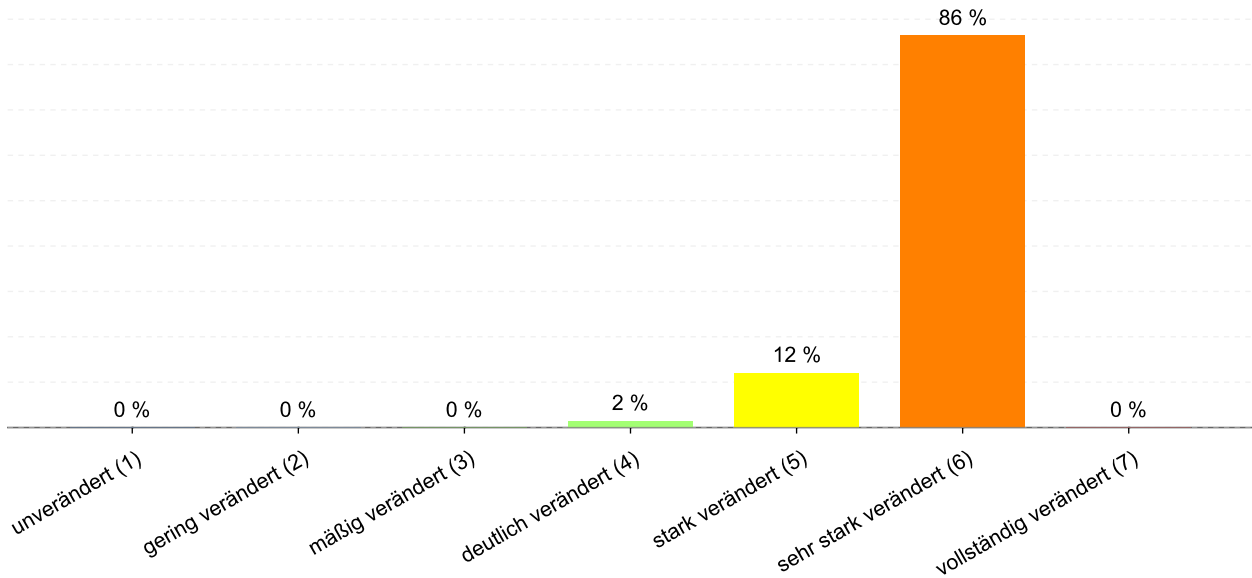
Abbildung 8: Anteil der Gewässerstrukturklassen im Wasserkörper DERW_DENW_2788812_0_7: Kettbach
