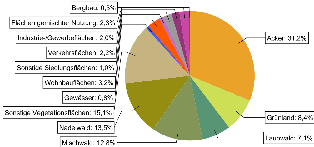
Abbildung 19: Landnutzung im Einzugsgebiet des Wasserkörpers DERW_DENW_278886_0_11: Kiffertbach, basierend auf ATKIS-Daten 2024. Landnutzungstypen mit weniger als 0,1% Anteil sind nicht dargestellt.
