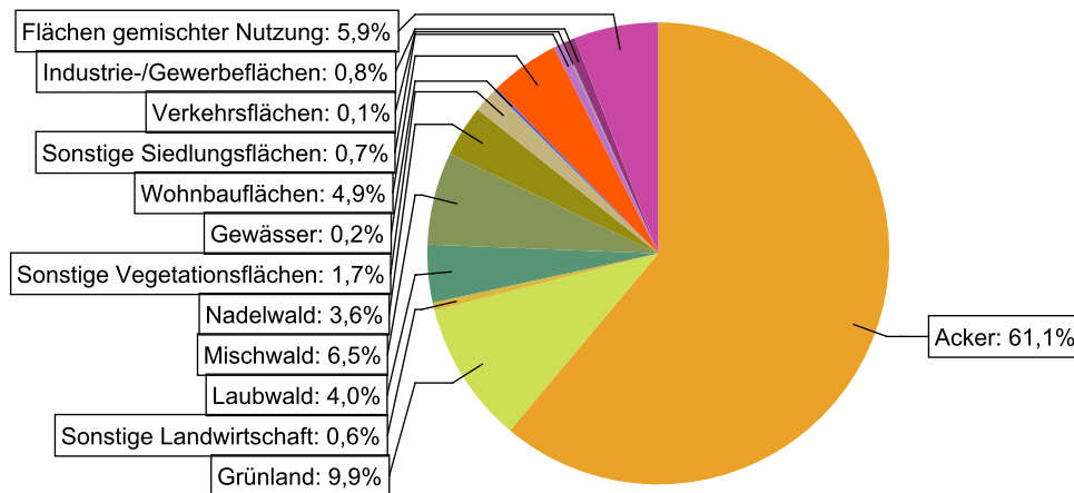
Abbildung 17: Landnutzung im Einzugsgebiet des Wasserkörpers DERW_DENW_2788842_0_14: Mühlenbach, basierend auf ATKIS-Daten 2024. Landnutzungstypen mit weniger als 0,1% Anteil sind nicht dargestellt.
