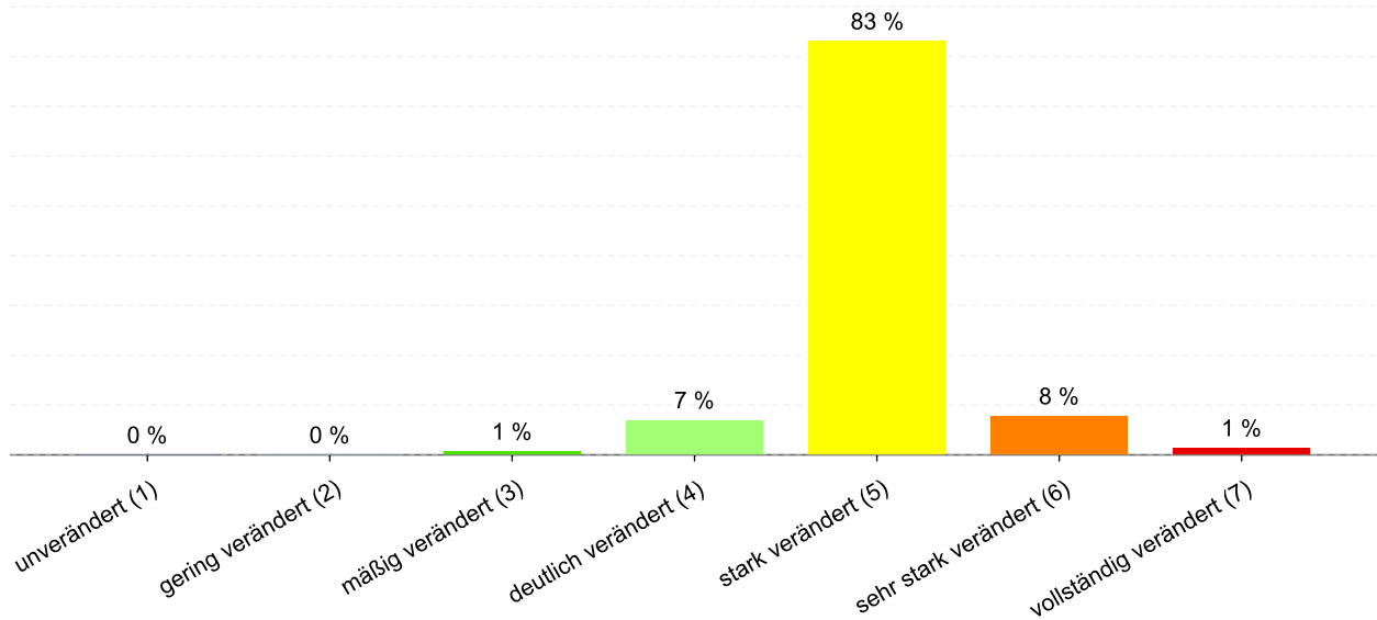
Abbildung 18: Anteil der Gewässerstrukturklassen im Wasserkörper DERW_DENW_2788842_0_14: Mühlenbach
