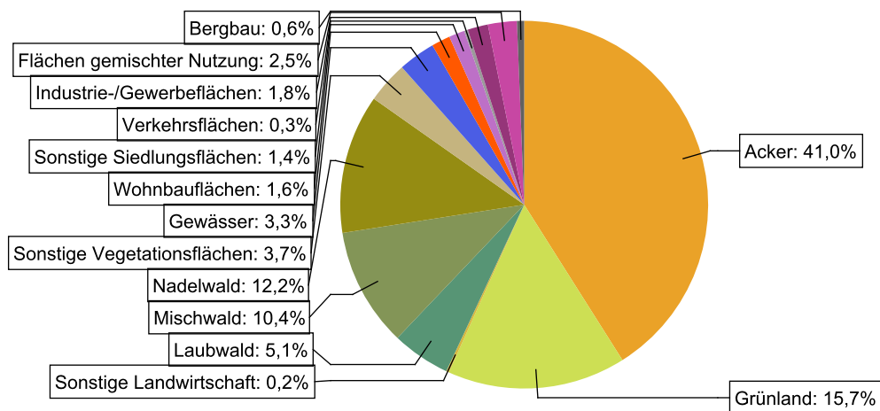
Abbildung 5: Landnutzung im Einzugsgebiet des Wasserkörpers DERW_DENW_27888_9_30: Heubach, basierend auf ATKIS-Daten 2024. Landnutzungstypen mit weniger als 0,1% Anteil sind nicht dargestellt.
