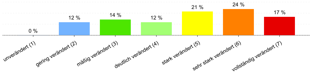
Abbildung 28: Anteil der Gewässerstrukturklassen im Wasserkörper DERW_DENW_2787664_5_9: Massener Bach
