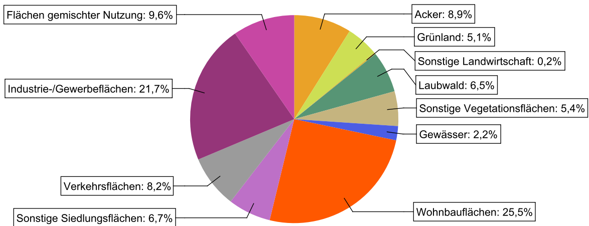
Abbildung 3: Landnutzung im Einzugsgebiet des Wasserkörpers DERW_DENW_286_90_93: Niers, basierend auf ATKIS-Daten 2024. Landnutzungstypen mit weniger als 0,1% Anteil sind nicht dargestellt.
