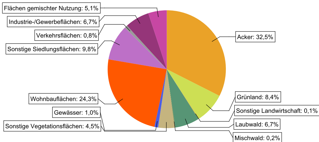
Abbildung 5: Landnutzung im Einzugsgebiet des Wasserkörpers DERW_DENW_286_93_101: Niers, basierend auf ATKIS-Daten 2024. Landnutzungstypen mit weniger als 0,1% Anteil sind nicht dargestellt.
