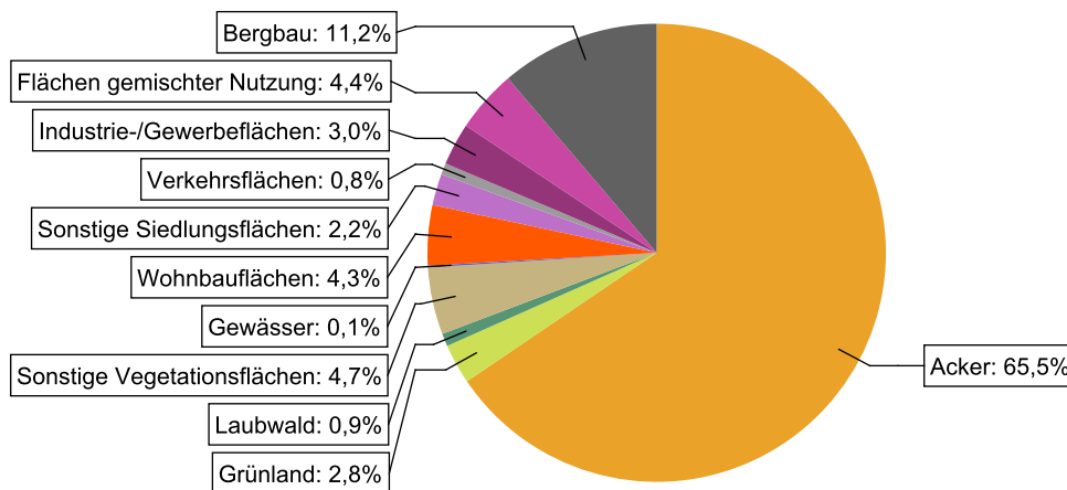
Abbildung 11: Landnutzung im Einzugsgebiet des Wasserkörpers DERW_DENW_286_111_114: Niers, basierend auf ATKIS-Daten 2024. Landnutzungstypen mit weniger als 0,1% Anteil sind nicht dargestellt.
