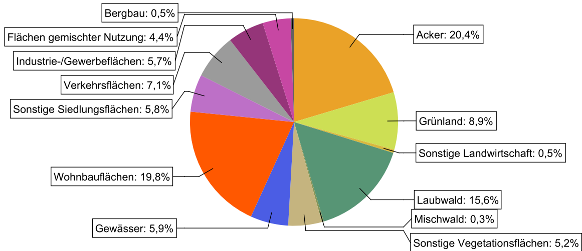
Abbildung 19: Landnutzung im Einzugsgebiet des Wasserkörpers DERW_DENW_286154_0_7: Cloer, basierend auf ATKIS-Daten 2024. Landnutzungstypen mit weniger als 0,1% Anteil sind nicht dargestellt.
