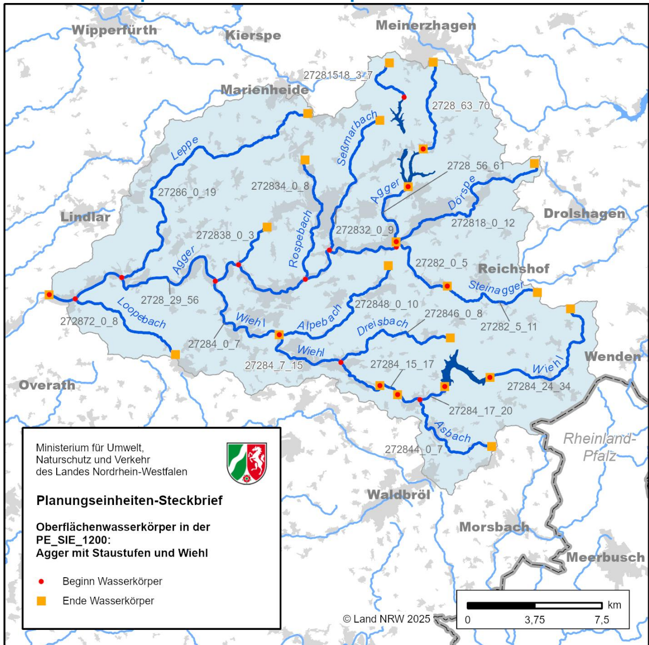
Abbildung 2: Oberflächenwasserkörper in der Planungseinheit PE_SIE_1200: Agger mit Staustufen und Wiehl
